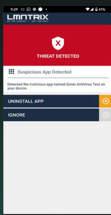
Malware
